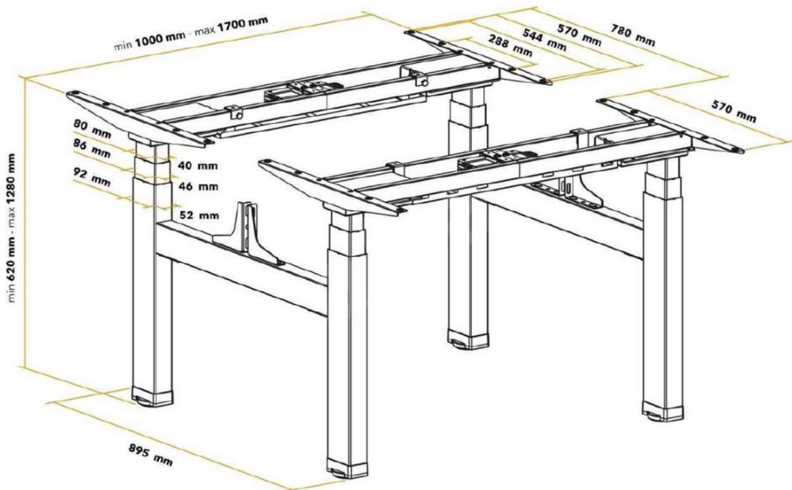
Nákres k položke č. 1 - Výškovo nastaviteľný pracovný stôl pre 2 miesta
