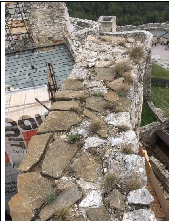
Súčasný stav koruny murív nad terasou – južná časť
