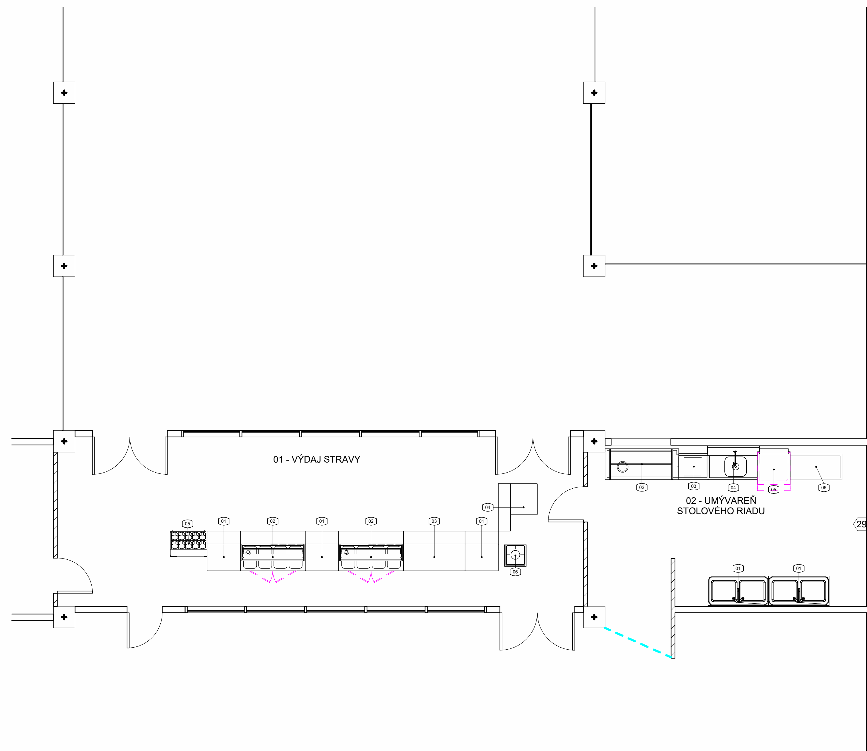
1 PODORYS 1NP 1 : 50
