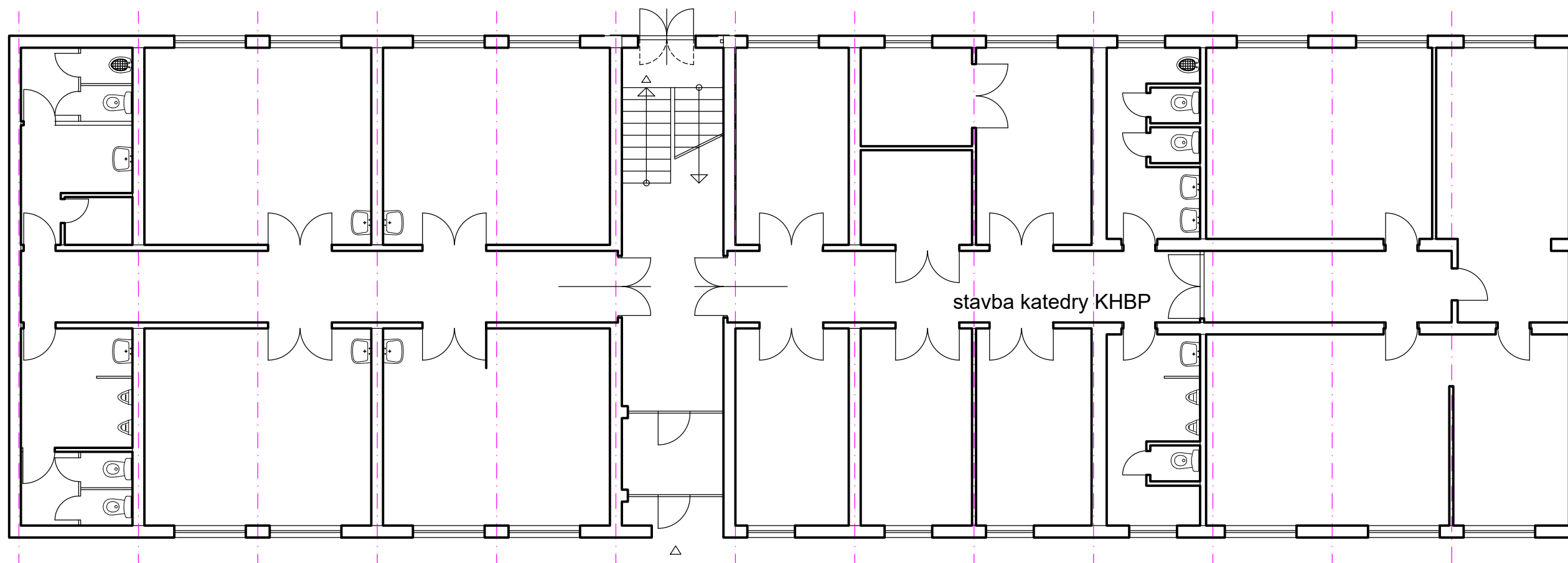
PODORYS - 1.NP
