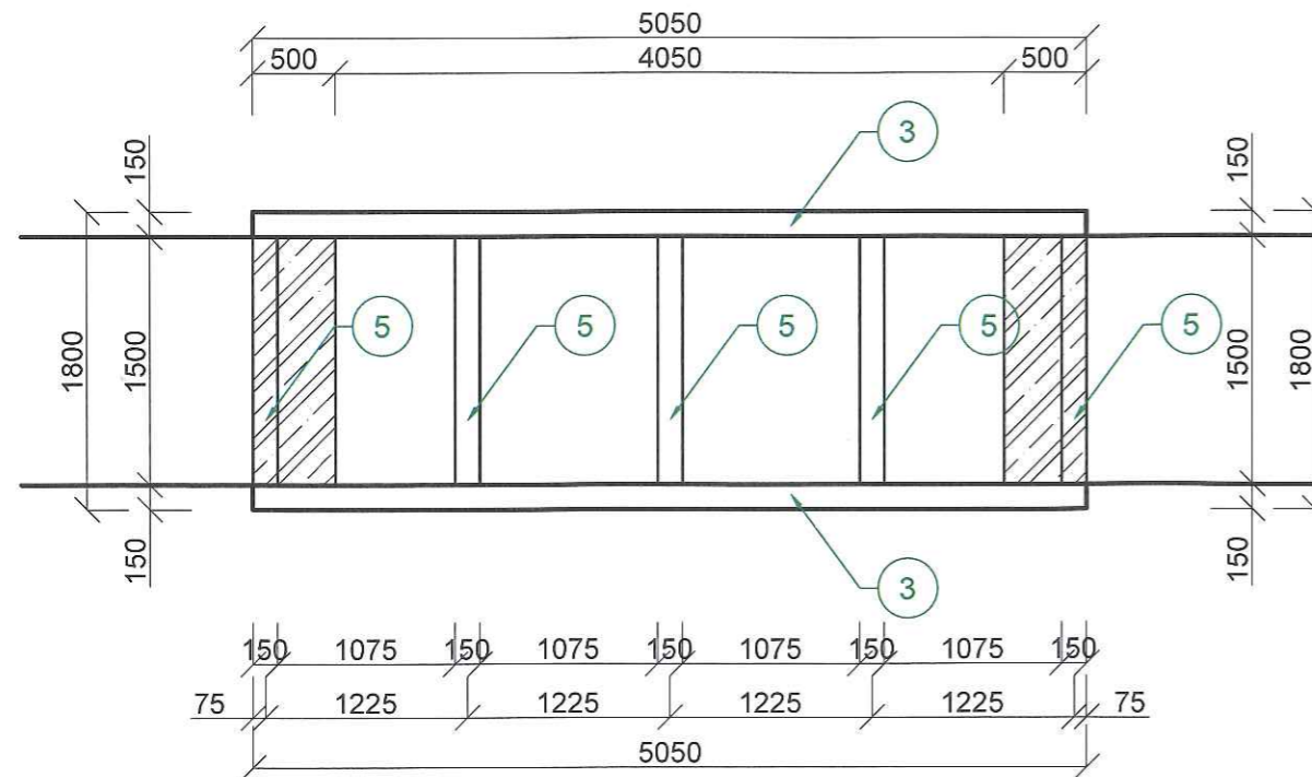
PÔDORYS 2 M1:50
