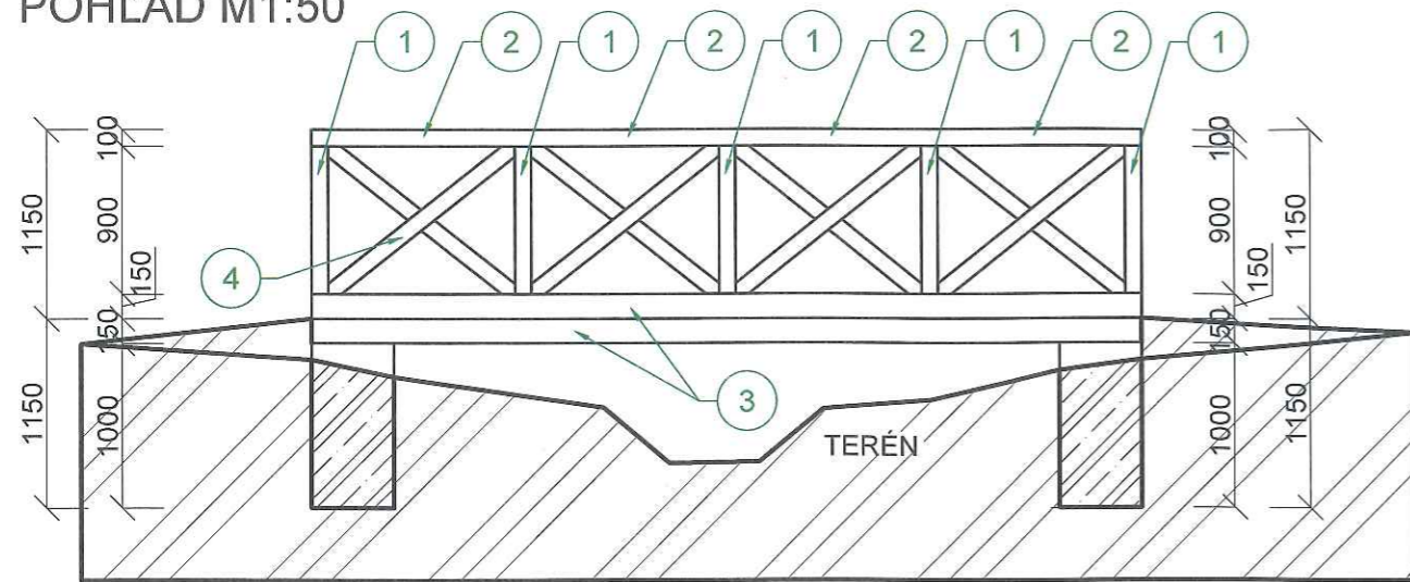
POHLAD M1:50
