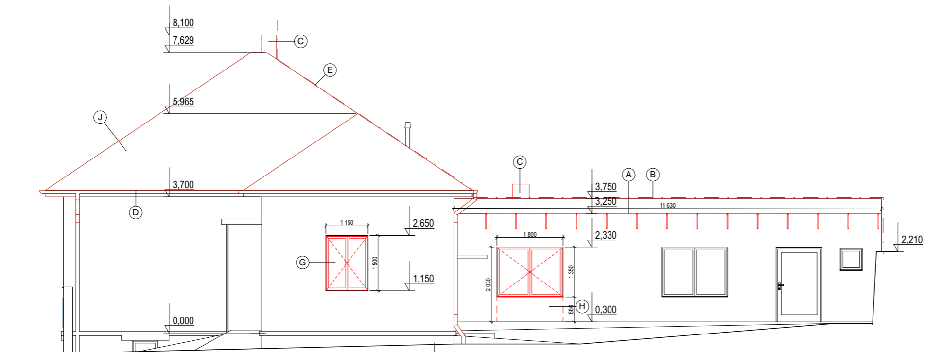
POHLAD PRAVÝ
