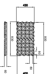
DETAIL ROŠTU
