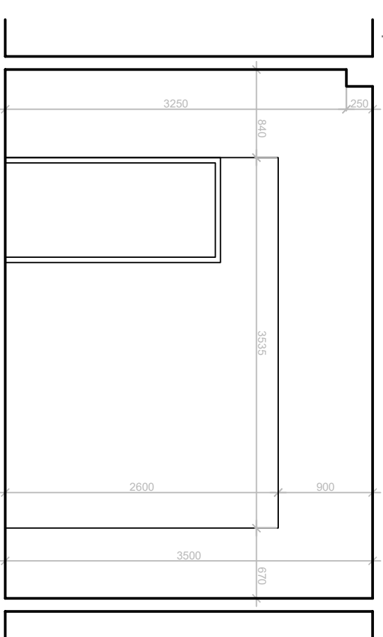
Rezopohľad - A-A'
