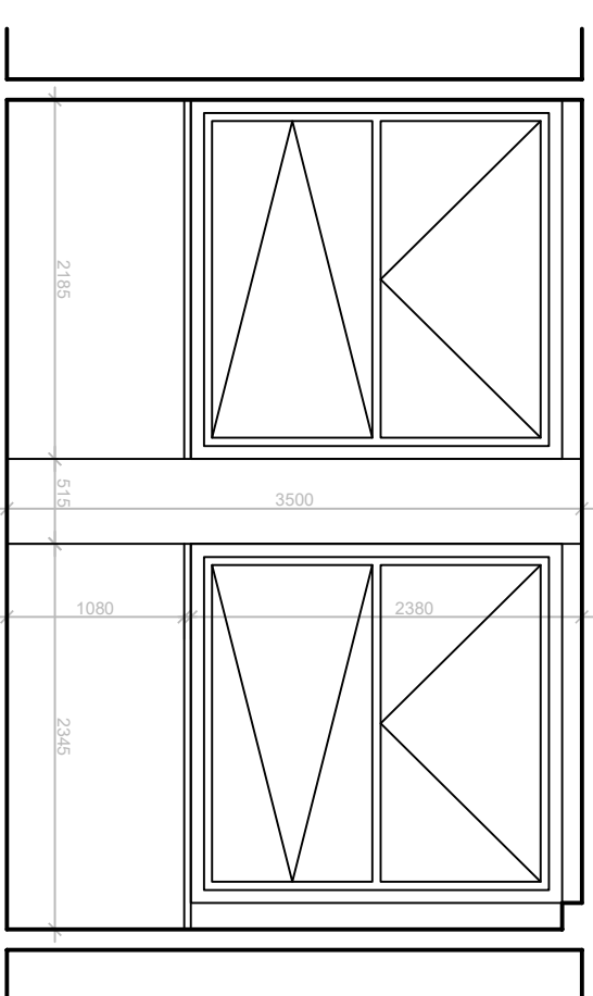
Rezopohľad - B-B'
