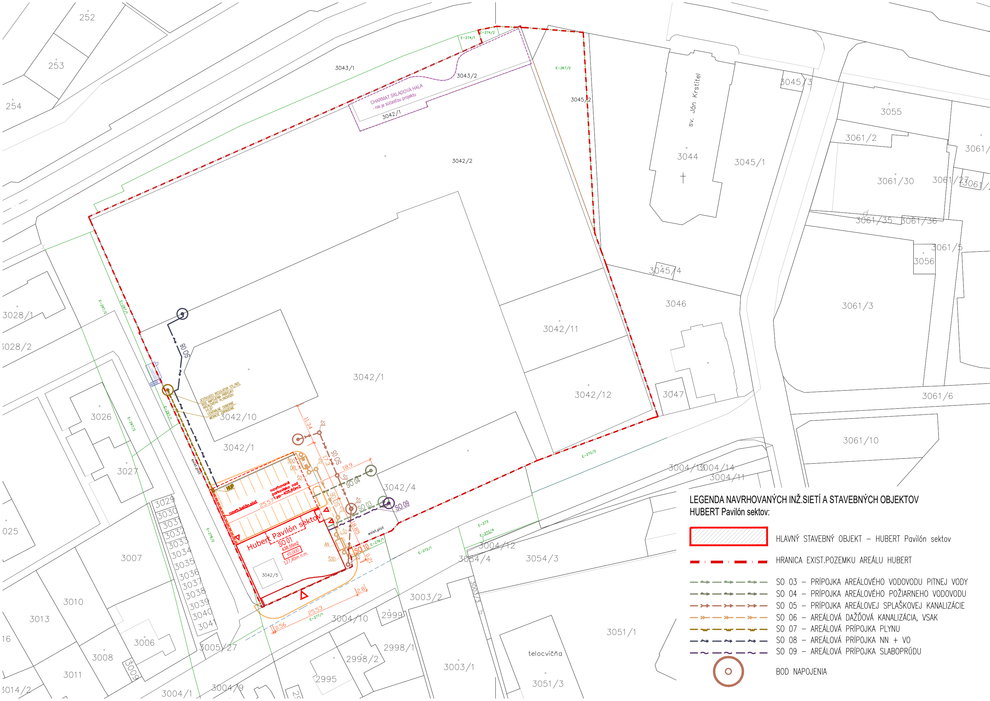
SITUÁCIA M1:500
