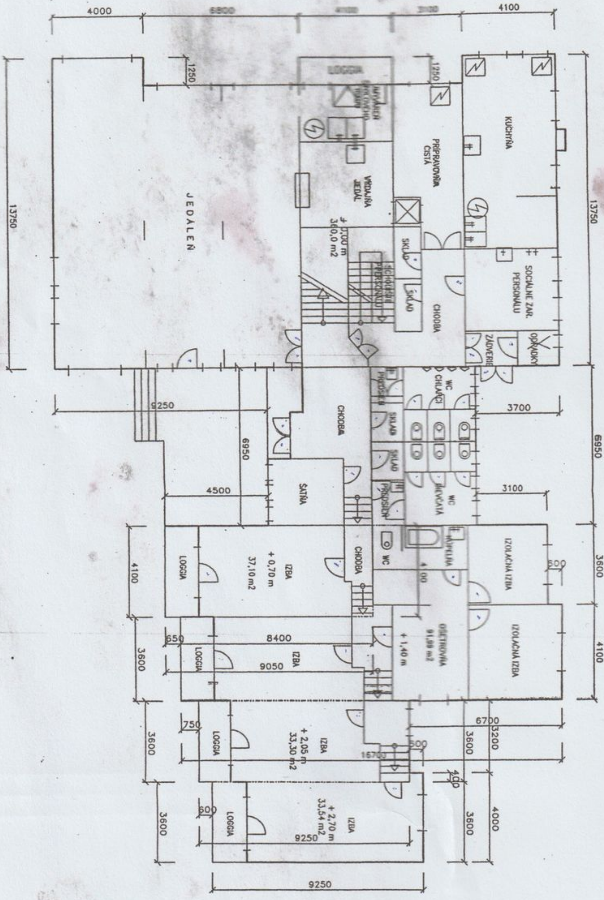
PIONIERSKY TABOR BIAZ SNV – RUIZIN PRÍZEMIE NA KÓTACH +0,00 + 0,70 + 1,40 + 2,05 + 2,70 m
