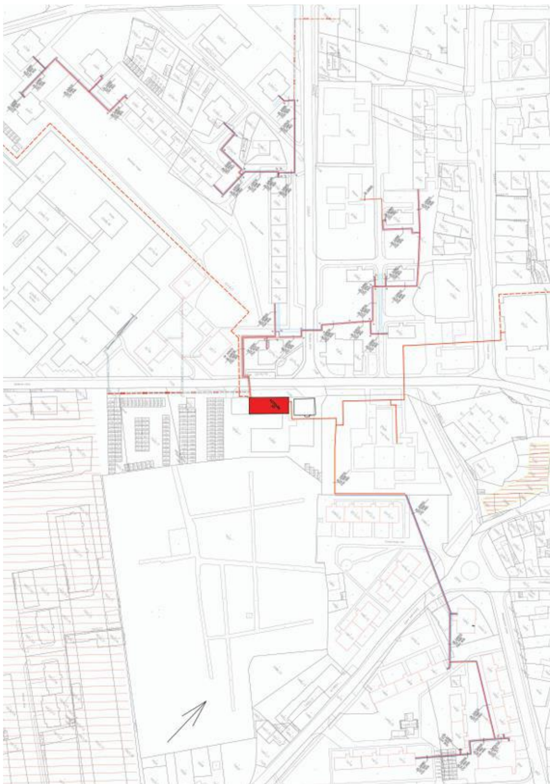
Obr. 1: Rozvody tepla – CZT Šamorín, K1
