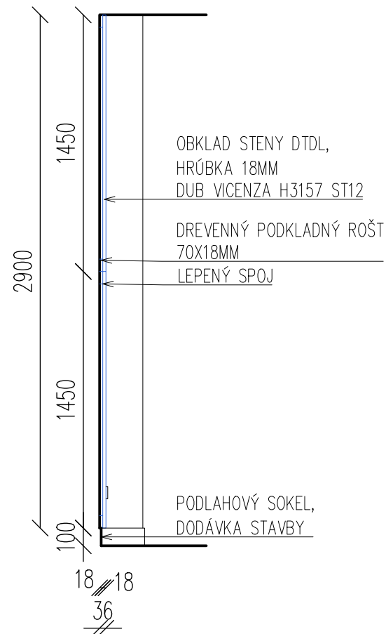
rez A-A'
