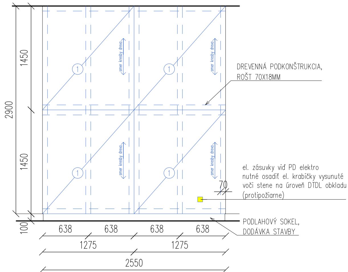
pohľad A
