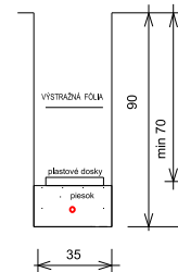
PRÍPOJKA NN REZ ULOŽENIA KÁBLA
