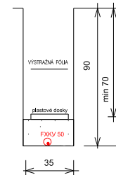
ROZVODY NN DPMB REZ ULOŽENIA KÁBLA
